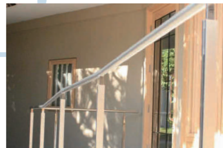
手摺 (特殊ブラスト・曲げ加工)
